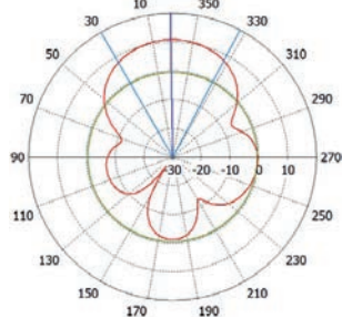
2,0 ГГц
