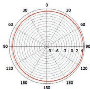
1,4 ГГц
