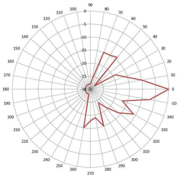
Диаграмма направленности на частоте 1.1 ГГц
