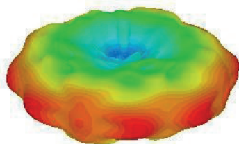
10 ГГц
