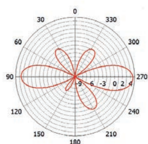
1,4 ГГц
