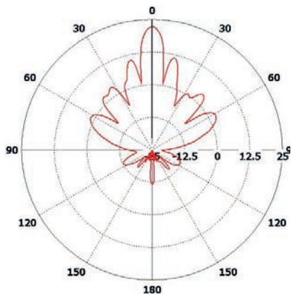
Вертикальная плоскость для порта H
