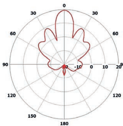
Вертикальная плоскость
