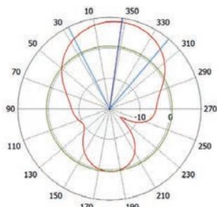
1,5 ГГц
