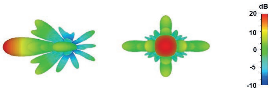
Вертикальная плоскость
