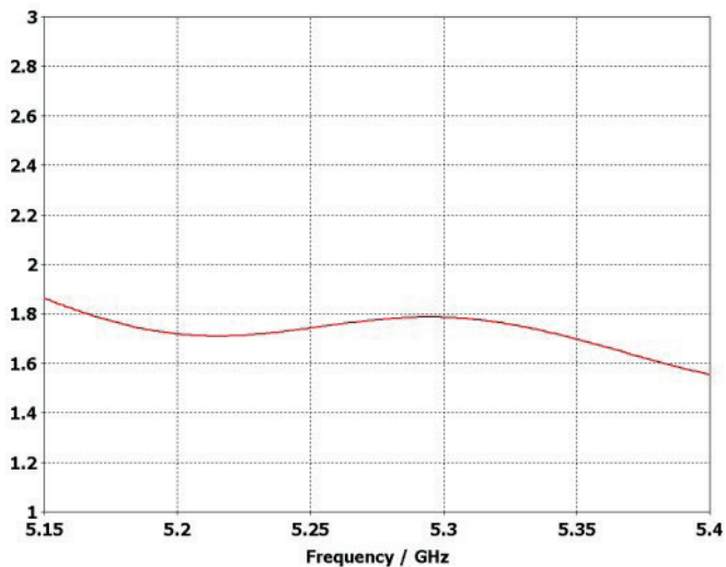
Порт H
