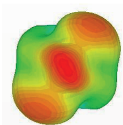
900 МГц
