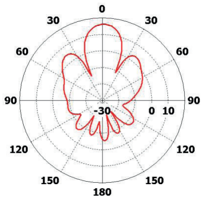
Вертикальная плоскость
