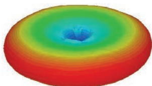
18 ГГц
