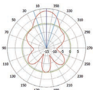
1,5 ГГц
