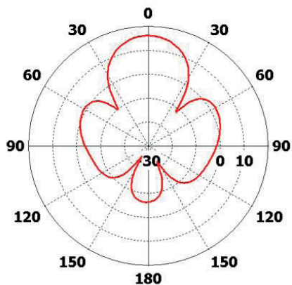
Горизонтальная плоскость
