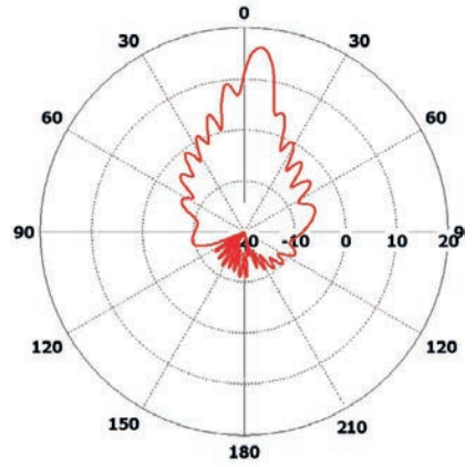
Вертикальная плоскость
