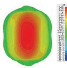
3 ГГц
