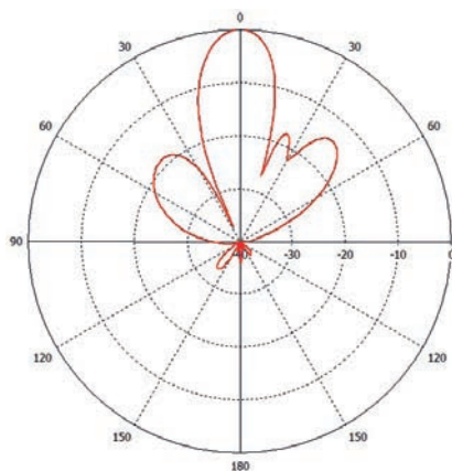
Вертикальная плоскость
