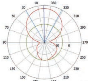
Горизонтальная плоскость
